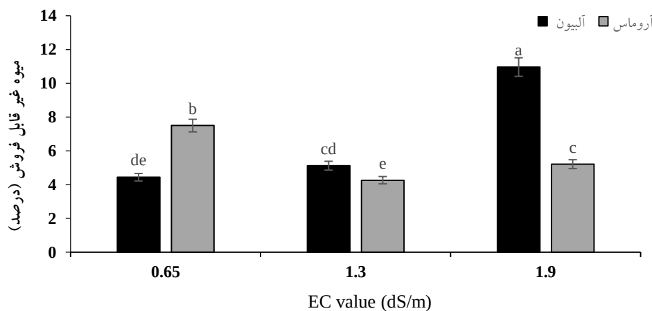
شکل ۳: تأثیر هدایت الکتریکی و رقم بر درصد میوه غیر قابل فروش در توت‌فرنگی در کشت بدون خاک در فضای آزاد
