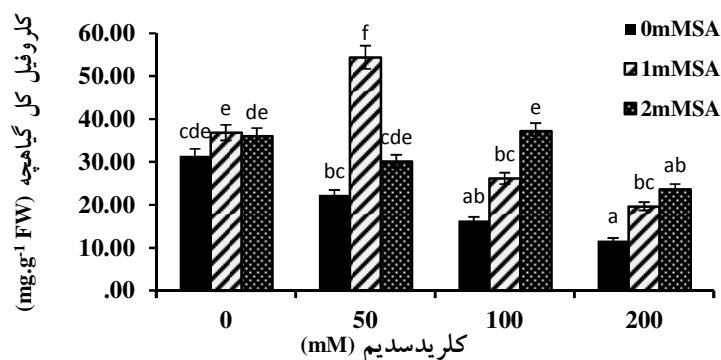
شکل ۶- تأثیر تنش شوری (غلظت ۰، ۵۰، ۱۰۰، ۲۰۰ میلی مولار) و سالیسیلیک اسید (غلظت ۰، ۱۰، ۲ میلی مولار) بر مقدار کلروفیل کل گیاهیچه شیرین بیان: حروف نامشابه نشان دهنده اختلاف معنی دار در سطح ۵٪ آزمون دانکن می باشد.
