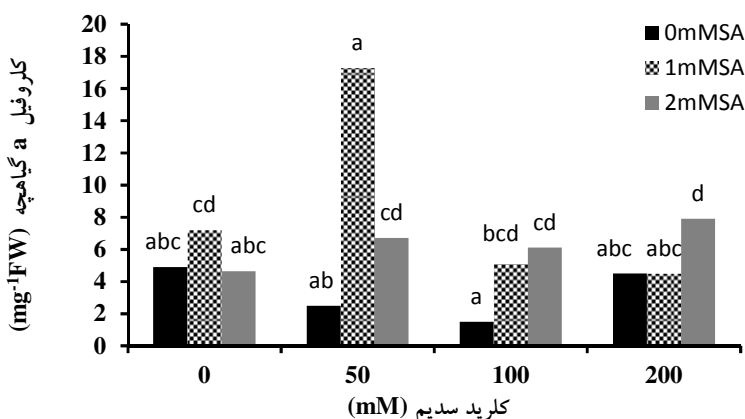
شکل ۴- تأثیر تنش شوری (غلظت ۰، ۵۰، ۱۰۰، ۲۰۰ میلی مولار) و اسیدیسیلیک اسید (غلظت ۰، ۱، ۲ میلی مولار) بر مقدار کلروفیل a گیاهچه شیرین بیان: حروف نامشابه نشان دهنده اختلاف معنی دار در سطح ۵٪ آزمون دانکن می باشد.
