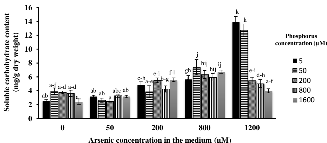
شکل ۲- اثر غلظت‌های مختلف آرسنیک و فسفر بر محتوی قندهای محلول بخش هوایی گیاه I. cappadocica حروف متفاوت هر ستون بیانگر معنی‌دار بودن اثر تیمارها بر میانگین قندهای محلول بخش هوایی گیاه، با استفاده از آزمون دانکن می‌باشد.
