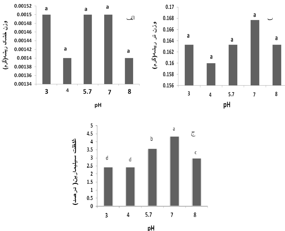
شکل ۵- مقایسه اثر pHهای مختلف محیط کشت مایع MS بر الف) وزن خشک، ب) وزن تر و ج) درصد سیلیمارین ریشه‌های در تولید شده در محیط کشت مایع. هر ستون نشان دهنده میانگین داده‌ها ± انحراف معیار است. ستون‌های دارای حداقل یک حرف مشترک با آزمون دانکن در سطح ۵ درصد تفاوت معنی‌داری با یکدیگر ندارند.
