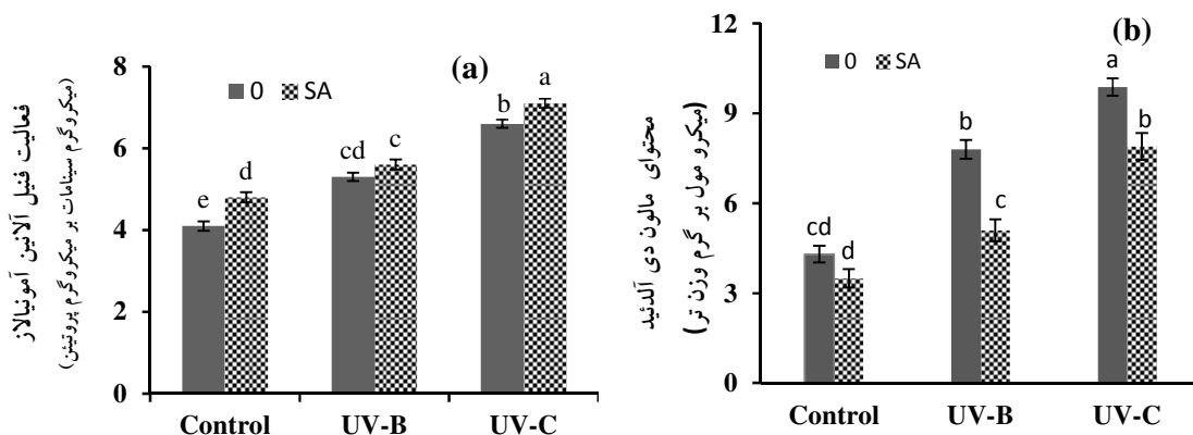
شکل ۶- تأثیر پرتوهای UV-B، UV-C و سالیسیلیک اسید بر محتوای فعالیت فنیل آلانین آمونیاژ (a) و محتوای مالون‌دی‌آلدئید (b) در گیاه بادرنجبویه. ۰ = بدون سالیسیلیک اسید و SA = به همراه سالیسیلیک اسید ۱ میلی‌مول. ستون‌ها نماینده میانگین سه تکرار و بارهای عمودی نشانگر انحراف استاندارد بوده و در هر ستون، میانگین‌های دارای حروف متفاوت دارای تفاوت معنی‌دار در سطح ۰/۰۵ با استفاده از آزمون دانکن هستند.
