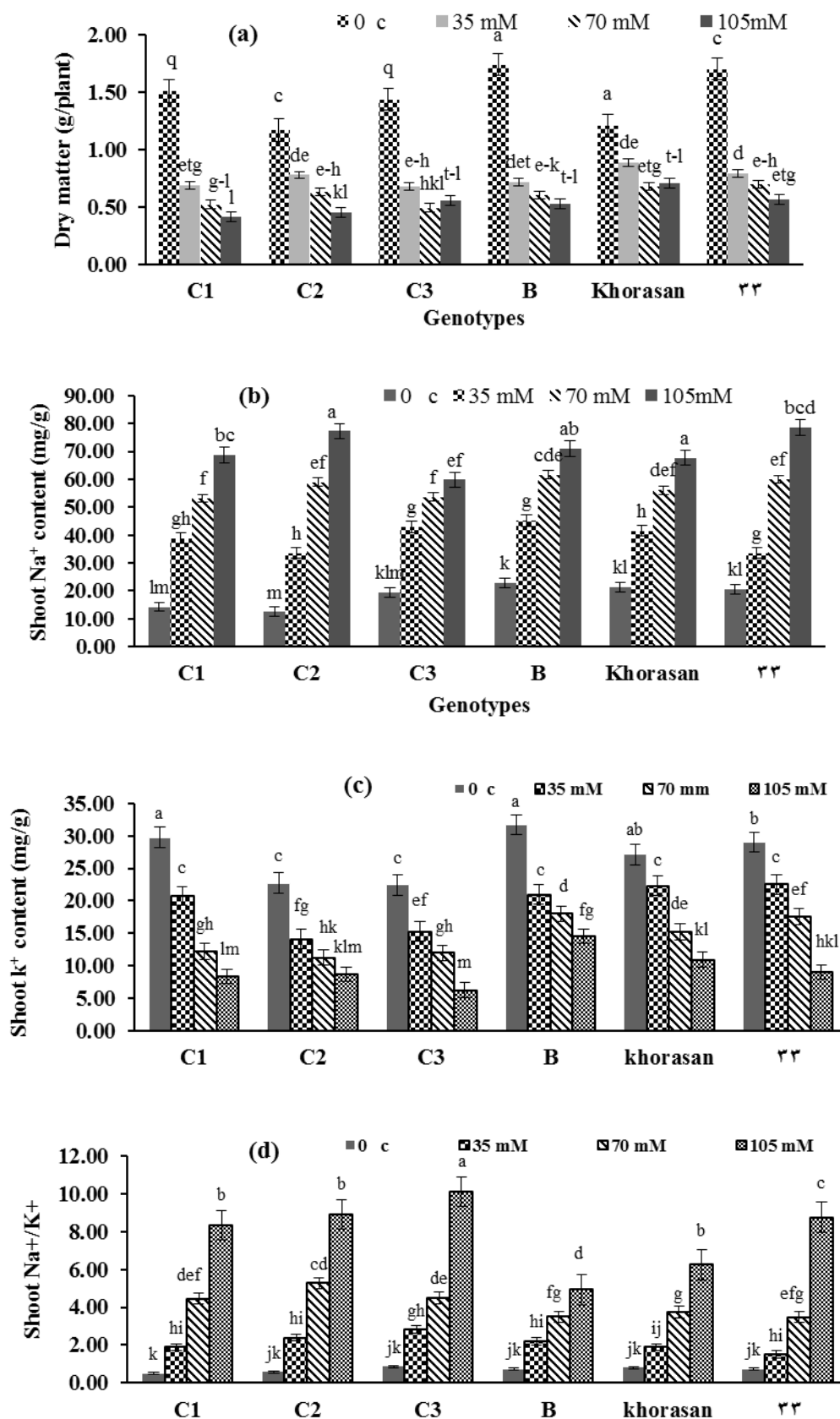
شکل ۱- بررسی میانگین اثر متقابل شوری و ژنوتیپ بر وزن خشک اندام هوایی (a)، سدیم (b)، غلظت پتاسیم (c) و نسبت سدیم به پتاسیم (d) در شش ژنوتیپ بزرگ. میانگین‌هایی که حداقل در یک حرف مشترک هستند فاقد تفاوت معنی دار آماری بر اساس آزمون حداقل تفاوت معنی دار در سطح ۵ درصد هستند.
