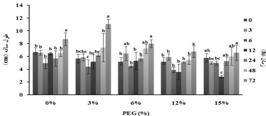
شکل ۹- تأثیر مقادیر مختلف PEG در زمان‌های مختلف روی طول ساقه در رقم Hyola308. حروف کوچک روی نمودار نشان‌دهنده مقایسه میانگین در هر سطح تنش است (آزمون دانکن و P \leq 0.01 ).
