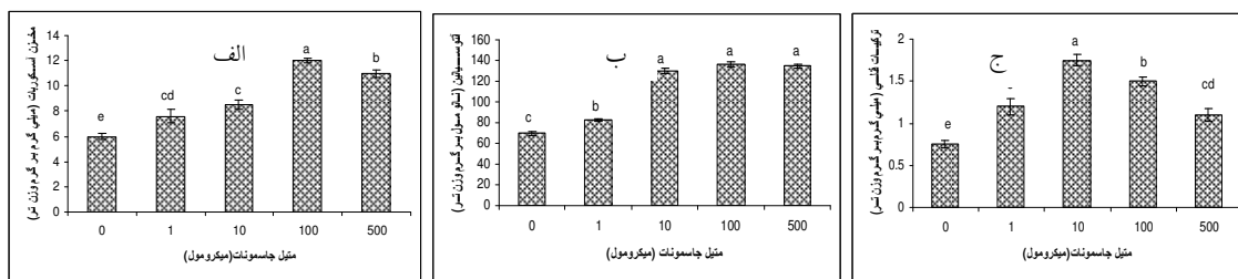
نمودار ۴- اثر متیل جاسمونات بر مقدار آسکوربات کل (مخزن آسکوربات) (الف)، ترکیبات فنلی (ب) و آنتوسیانین (ج) در گیاه سویا در مرحله رویشی (مقادیر میانگین ۳ تکرار می باشد و حروف یکسان بیانگر عدم اختلاف معنی دار با استفاده از آزمون دانکن می باشد).
