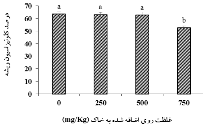
شکل ۱- تأثیر سمیت روی بر درصد کلوروفیل ریشه. میانگین‌های دارای حروف مشابه از نظر آماری تفاوت معنی داری در سطح احتمال پنج درصد ندارند.
