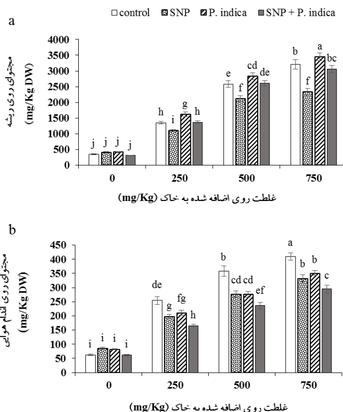
شکل ۲- مقایسه میانگین برهمکنش روی، قارچ P. indica و محلول پاشی برگه نیتروپروساید سدیم (SNP) بر محتوای روی ریشه (a) و اندام هوایی (b). میانگین‌های دارای حروف مشابه از نظر آماری تفاوت معنی‌داری در سطح احتمال پنج درصد ندارند.
