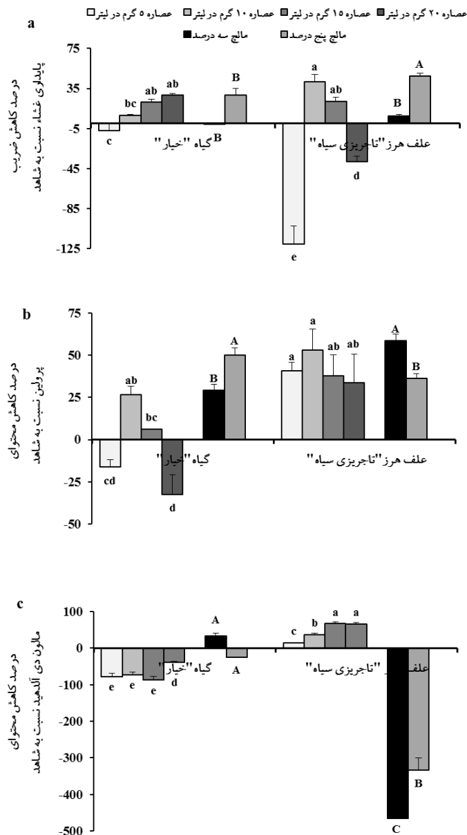
شکل ۲- تأثیر دو نوع تیمار عصاره آبی و مالچ‌برگی اکالیپتوس ( E. globulus ) بر درصد کاهش ضریب پایداری غشا (a)، محتوا پرولین (b)، محتوا مالون دی‌آلدئید (c) گیاهچه‌های خیار ( Cucumis sativus var. beith alpha ) و علف هرز تاجریزی سیاه ( Solanum nigrum ) داده-ها میانگین سه تکرار \pm خطای معیار هستند (براساس آزمون دانکن، تفاوت معنی‌داری ( P \leq 0.05 ) بین میانگین‌های واجد حرف یا حروف یکسان وجود ندارد). واحد اندازه‌گیری میکرومول بر گرم وزن تر نمونه است.
