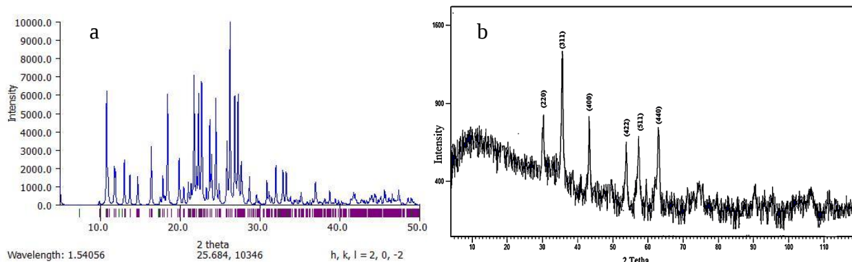
شکل ۳- الگوی XRD کمپلکس آهن (a) و نانو ذرات آهن (b)
