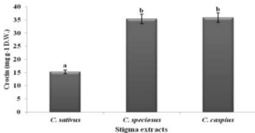
شکل ۱- محتوای کروسین در کللاه سه گونه خزری، زیبا و زراعی زعفران. حروف متفاوت نشان دهنده وجود اختلاف معنی‌دار در سطح ۵ درصد آزمون توکی هستند ( P \leq 0.05 ).
