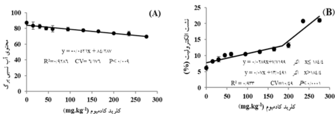
شکل ۳- روند تغییرات محتوی آب نسبی برگ (A) و میزان نشت الکترولیت (B) گیاه دارویی خرفه در پاسخ به افزایش غلظت کادمیوم خاک با استفاده از مدل خطی (رابطه ۵) و دوتکه‌ای (رابطه ۶). میله‌ها نشان‌دهنده خطای استاندارد (SE) و N=۳ است.
