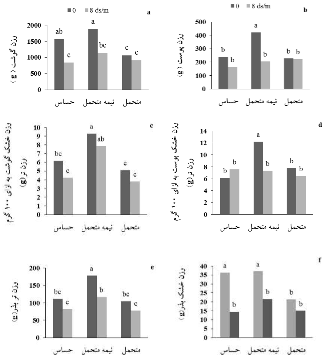
شکل ۲- اثر متقابل سطوح شوری و توده‌ها بر وزن تر گوشت (a) و وزن تر پوست میوه (b)، وزن خشک به ازای ۱۰۰ گرم تر گوشت (c) و وزن خشک به ازای ۱۰۰ گرم تر پوست میوه (d)، وزن تر بذری (e) و وزن خشک بذری (f). متحمل (آناناسی)، نیمه‌متحمل (سبز اصفهان) و حساس به شوری (گنگی). ستون‌هایی که در یک حرف متفاوت هستند دارای تفاوت معنی‌دار در سطح ۵ درصد براساس آزمون LSD می‌باشند.
