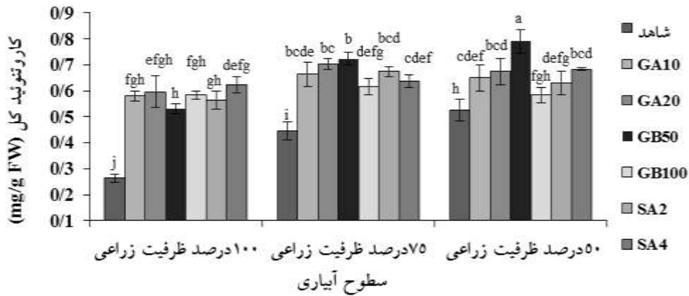
شکل ۲- اثر متقابل تنش کم آبی و سالیسیلیک اسید (SA)، گلیاسین بتائین (GB)، گاما آمینوبوتیریک اسید (GA) بر میزان کاروتنوئید کل. ستون‌های دارای حروف مشابه نشان‌دهنده عدم اختلاف معنی‌دار بین تیمارها است.
