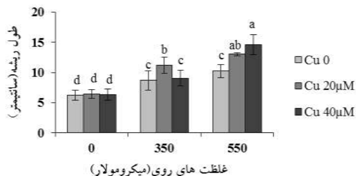
شکل ۱- مقایسه برهمکنش غلظت های سولفات روی و سولفات مس بر روی طول ریشه گیاه ریحان ( Ocimum basilicum ). داده ها میانگین سه تکرار ± خطای استاندارد (SE) است و حروف نامشابه نشان دهنده اختلاف معنی دار بر اساس آزمون دانکن ( P < 0.05 ) است.
