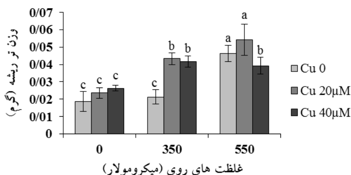
شکل ۳- مقایسه برهمکنش غلظت های سولفات روی و سولفات مس بر وزن تر ریشه گیاه ریحان ( Ocimum basilicum ). داده ها میانگین سه تکرار ± خطای استاندارد (SE) است و حروف نامشابه نشان دهنده اختلاف معنی دار بر اساس آزمون دانکن ( P < 0.05 ) است.
