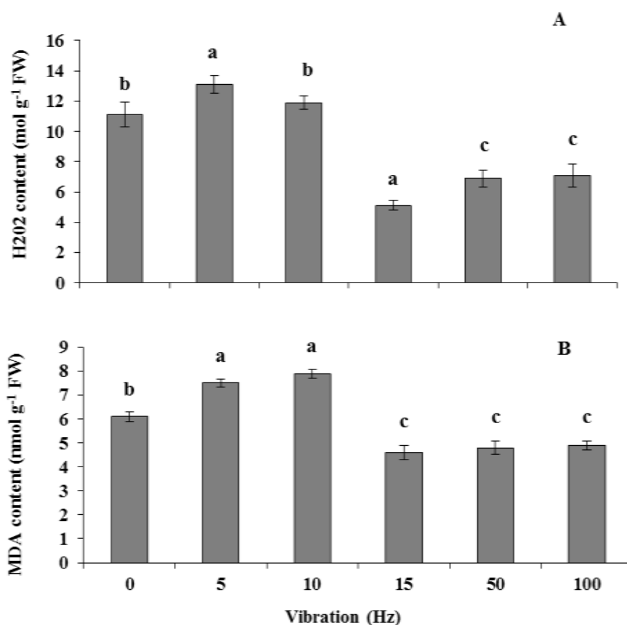
شکل ۲- تأثیر ارتعاشات سینوسی بر محتوای H 2 O 2 (A) و مالون دی آلدئید (B) در بابونه گیلانی. مقادیر میانگین ± تکرار ۴ ± انحراف معیار و حروف نامشابه بیانگر اختلاف معنی دار بر اساس آنالیز واریانس یکطرفه می باشد (P ≤ ۰/۰۵).
