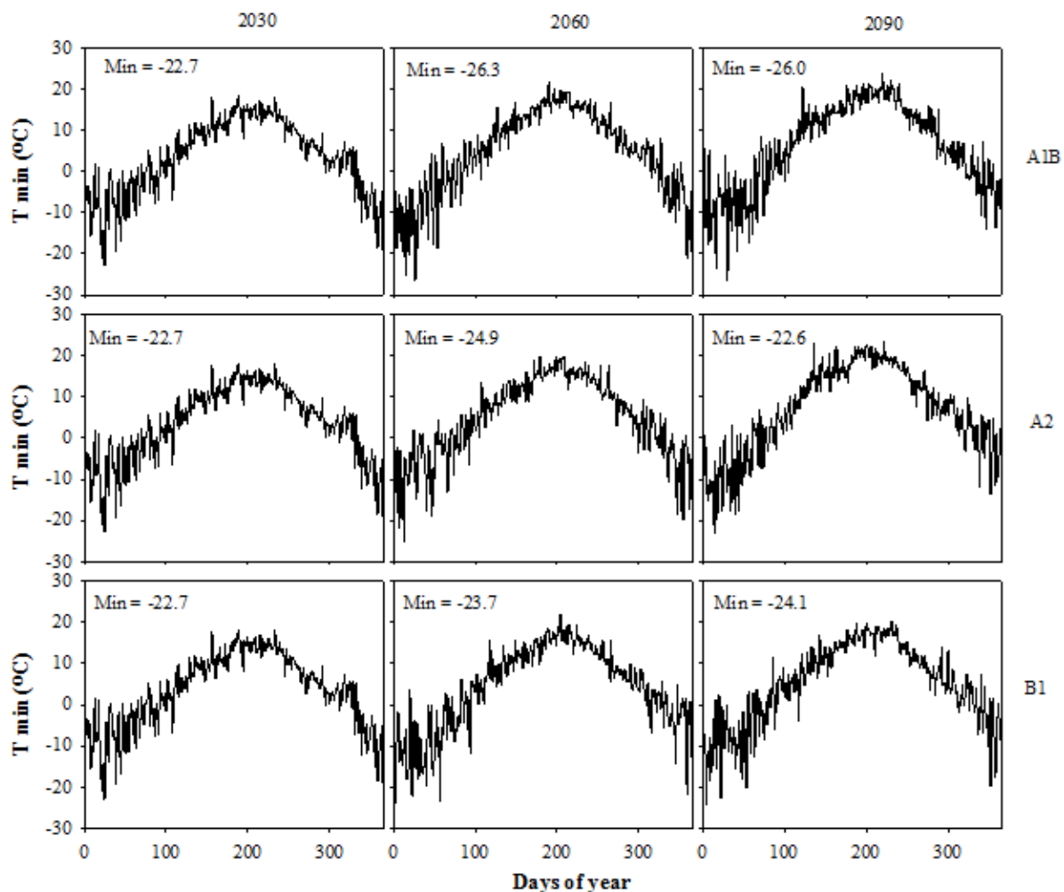
شکل ۷- روند تغییرات دمای کمینه در طول سال و کمترین دمای کمینه پیش‌بینی شده (min) در سناریوهای مختلف تغییر اقلیم برای سه دوره زمانی ۲۰۳۰، ۲۰۶۰ و ۲۰۹۰ در مدل گردش عمومی HadCM3.
