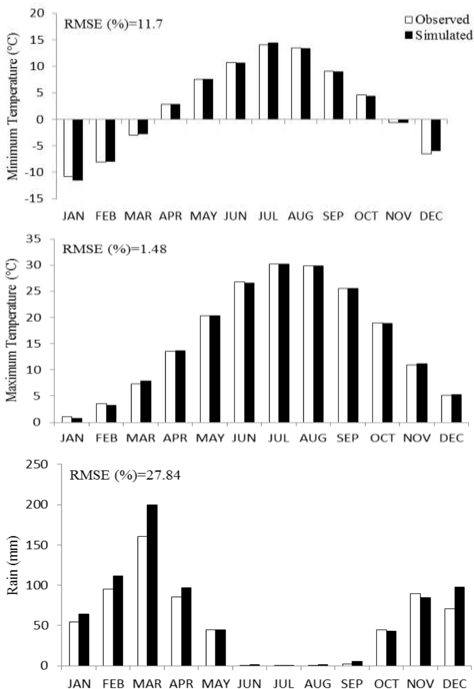
شکل ۲- اختلاف بین داده‌های اقلیمی (دمای بیشینه و کمینه و بارندگی) مشاهده شده و پیش‌بینی شده توسط مدل LARS-WG و تعیین اعتبار داده‌های اقلیمی با استفاده از RMSE.
