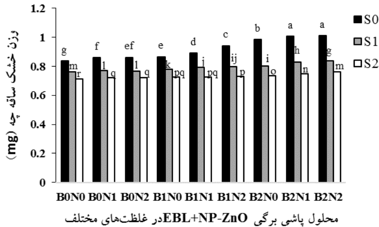
شکل ۵- شاخص وزن خشک ساقه‌چه بذرهاى گوجه‌فرنگی متأثر از محلول پاشی EBL+NP-ZnO و تنش شوری. حروف مشابه بیانگر عدم اختلاف معنی‌دار در سطح احتمال ۵ درصد می‌باشد (LSD= ۰/۰۰۶۴).
