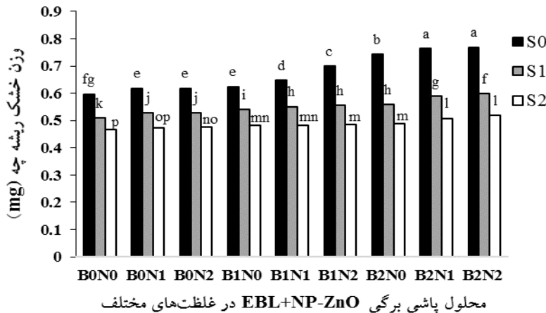
شکل ۴- شاخص وزن خشک ریشه‌چه بذرهاى گوجه‌فرنگی متأثر از محلول پاشی EBL+NP-ZnO و تنش شوری. حروف مشابه بیانگر عدم اختلاف معنی‌دار در سطح احتمال ۵ درصد می‌باشد (LSD= ۰/۰۰۷۷).
