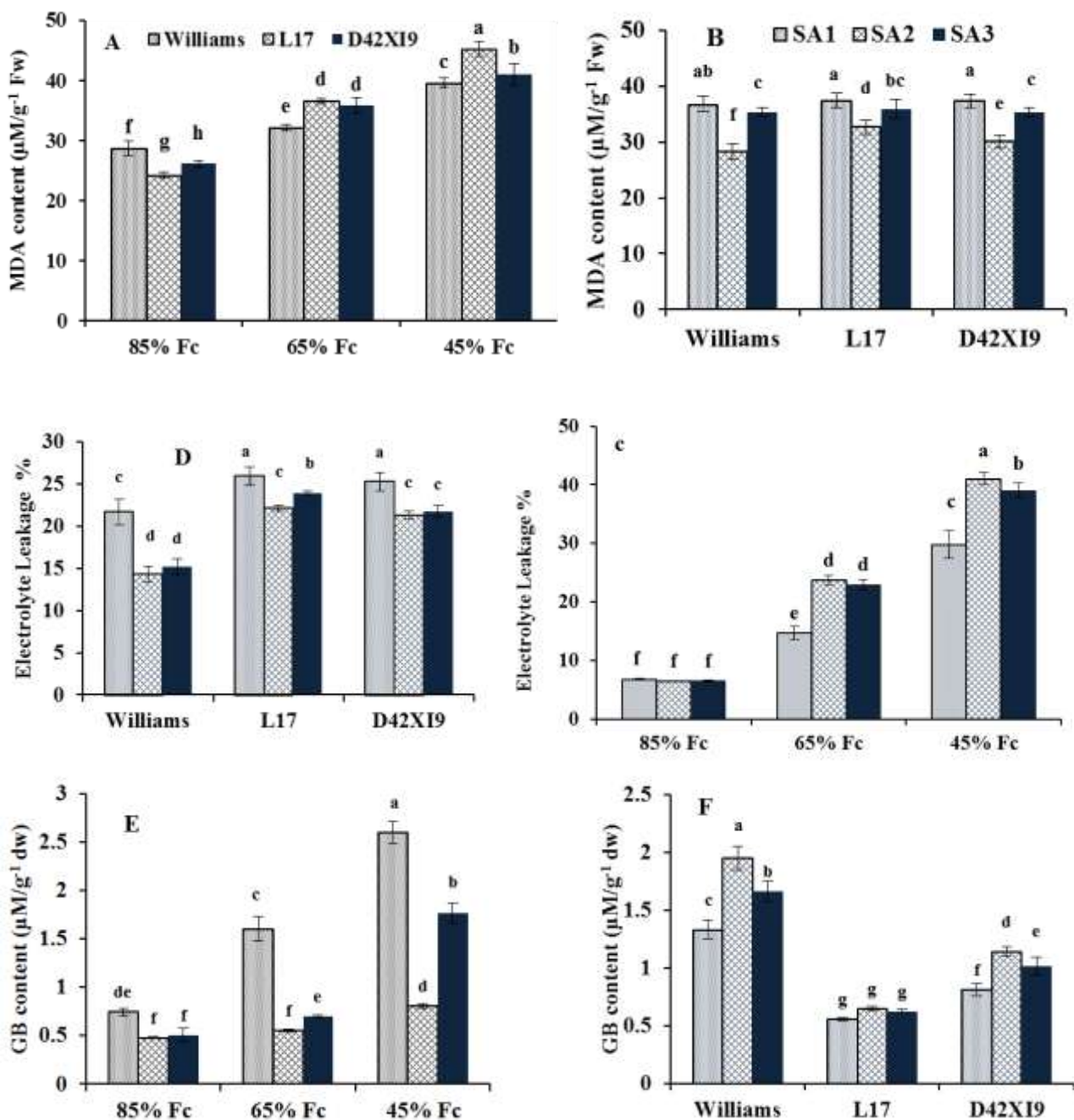
شکل ۱- اثر برهمکنش رژیم آبیاری و ژنوتیپ‌های سویا (A-C-E) و ژنوتیپ و غلظت‌های سالیسیک اسید (B-D-F) بر میزان فعالیت مالون دآلدئید، نشن کترولیتی و میزان گلاسیسین بتائین، داده‌ها میانگین سه تکرار \pm SE می‌باشد.
