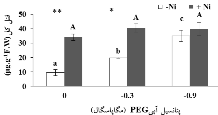
شکل ۶- اثر نیکل بر محتوای فنل کل گیاه F. garcinii تحت تنش خشکی حاصل از PEG 6000 (میانگین سه تکرار ± خطای استاندارد). حروف غیرمشترک، بیانگر اختلاف معنی دار بین تیمارها براساس آزمون Duncan ( P < 0.05 ) است. علامت * و ** به ترتیب نشان دهنده تفاوت معنی دار در سطح ۵ و ۱ درصد بین دو تیمار دارا و فاقد نیکل است.
