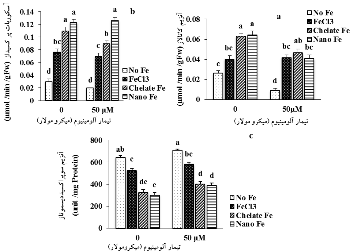
شکل ۲- مقایسه میانگین اثر متقابل اشکال مختلف آهن و آلومینیوم بر میزان فعالیت آنزیم‌های کاتالاز (a)، آسکوربات پراکسیداز (b) و سوپراکسیددیس‌موتاز (c) در گیاه بادرنجبویه. (مقادیر میانگین سه تکرار ± انحراف معیار می‌باشند. ستون‌های نشان داده شده با حروف متفاوت در سطح P \leq 0.05 اختلاف معنی‌داری دارند)
