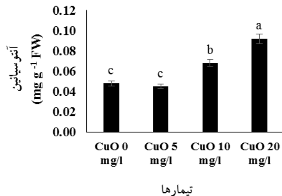
شکل ۵- تأثیر سطوح مختلف نانوذرات اکسید مس (CuO) بر مقدار آنتوسیانین (میلی گرم بر گرم وزن تر) گیاه نعناع‌فلغلی. حروف مشابه نشان‌دهنده عدم وجود اختلافات معنی‌دار در سطح P < 0/05 است.
