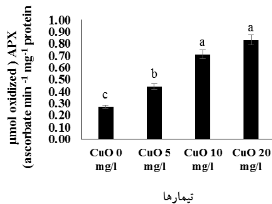
شکل ۹- تأثیر سطوح مختلف نانوذرات اکسید مس (CuO) بر فعالیت آسکوربات پراکسیداز (میکرومول آسکوربات اکسید شده در دقیقه بر میلی گرم پروتئین) نعنای فلفلی. حروف مشابه نشان دهنده عدم وجود اختلافات معنی دار در سطح P < 0.05 است.
