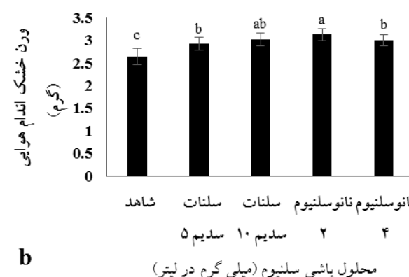
شکل ۱- اثر ساده تنش شوری (a) و محلول پاشی سلنیوم (b) بر وزن خشک اندام هوایی بادنجنبویه. حروف لاتین مشابه به معنی عدم تفاوت معنی دار در آزمون دانکن است. بارهای روی نمودار خطای استاندارد است.
