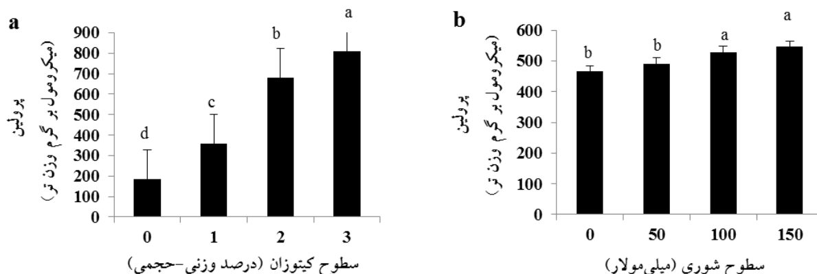
شکل ۳- مقایسه میانگین اثرات ساده کیتوزان (a) و شوری (b) بر روی پروئین در گلرنگ. حروف متفاوت در هر ستون نشان دهنده تفاوت معنی دار در سطح احتمال ۵ درصد بر حسب آزمون دانکن است.
