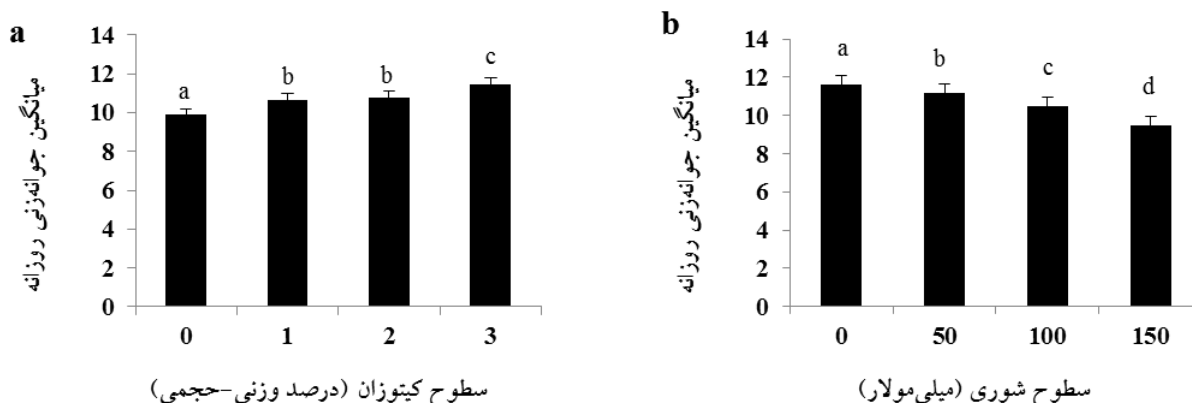
شکل ۲- مقایسه میانگین اثرات ساده کیتوزان (a) و شوری (b) بر روی میانگین جوانه زنی روزانه در گلرنگ. حروف متفاوت در هر ستون نشان دهنده تفاوت معنی دار در سطح احتمال ۵ درصد بر حسب آزمون دانکن است.
