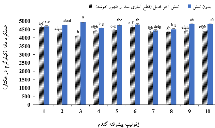
شکل ۱۰- مقایسه میانگین اثر متقابل تشنش × ارقام برای صفت عملکرد دانه. حروف یکسان بیانگر عدم اختلاف معنی دار در سطح P \leq 0.05 است.
