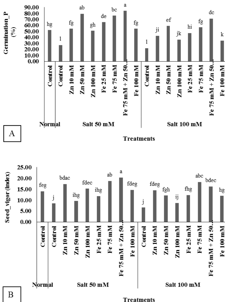
شکل ۲- تأثیر پرایمینگ ریزمغذی‌های آهن و روی و تنش شوری بر درصد جوانه‌زنی (A) و بیه بذر (B) شاهدانه. حروف غیرمشابه گویای وجود اختلافات معنی‌دار در سطح P < 0.05 است.
