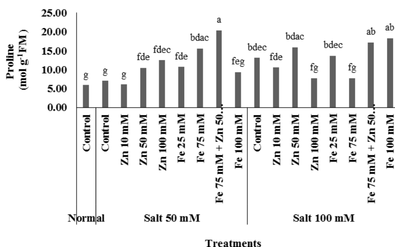
شکل ۵- تأثیر پرایمینگ ریزمغذی‌های آهن و روی و تنش شوری بر محتوی پرولین در گیاه شاهدانه. حروف غیرمشابه گویای وجود اختلافات معنی‌دار در سطح P < 0.05 است.
