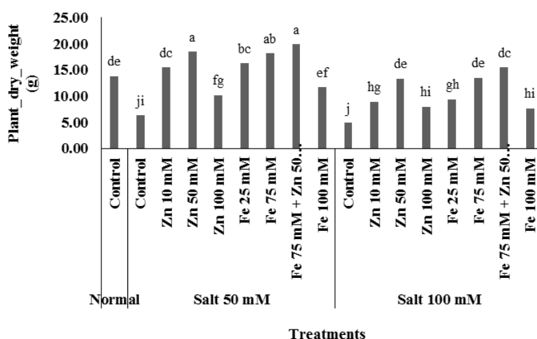
شکل ۳- تأثیر پرایمینگ ریزمغذی‌های آهن و روی و تنش شوری بر وزن خشک بوته گیاه شاهدانه. حروف غیرمشابه گویای وجود اختلافات معنی‌دار در سطح P < 0.05 است.
