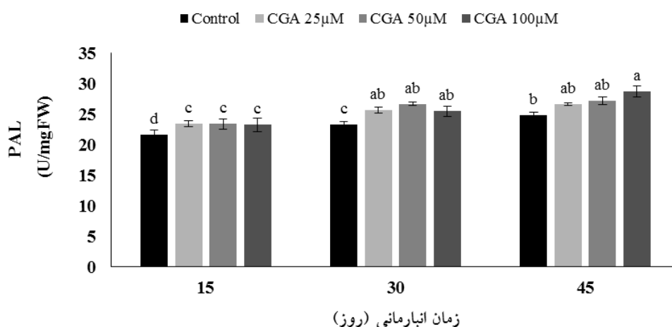
شکل ۷- تأثیر تیمار کلروژنیک اسید بر فعالیت آنزیم فنیل آلانین آمونیالیاز طول انبارمانی در دمای ۱ درجه سانتی گراد به مدت ۴۵ روز. خطوط عمودی بیانگر خطای استاندارد است.
