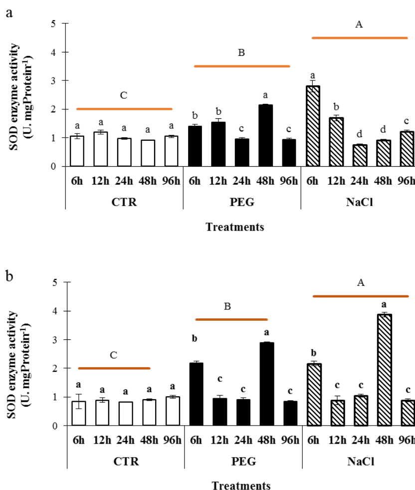
شکل ۱- تأثیر تنش اسمزی (PEG) و شوری (NaCl) بر میزان فعالیت آنزیم سوپراکسید دیسموتاز (SOD) در بافت‌های اندام‌هوایی (a) و ریشه (b) گیاه کنبجد طی بازه‌های مختلف (۶، ۱۲، ۲۴، ۴۸، ۹۶ ساعت) پس از اعمال تنش. CTR نشان‌دهنده تیمار شاهد در بازه‌های زمانی مختلف است. مقایسه میانگین‌های اثرات ساده بین تنش‌ها با حروف لاتین بزرگ نشان داده شده است. حروف مشترک نشان‌دهنده عدم اختلاف معنی‌دار بین تیمارها با استفاده از آزمون LSD ( P < 0.01 ) است.
