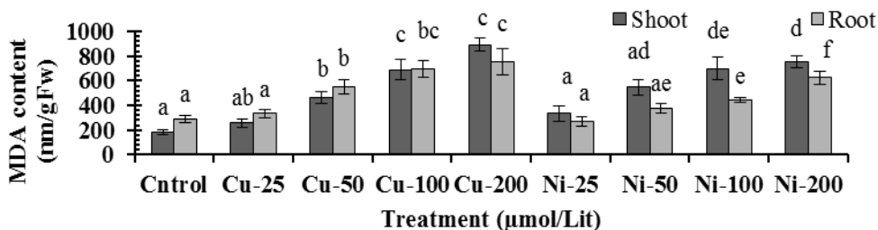
شکل ۳- مقایسه‌ی میانگین ۳ تکرار \pm SE MDA در اندام هوایی و ریشه نمونه‌های شاهد و تیمارهای مختلف مس و نیکل. مقایسه‌ی میانگین داده‌ها با آزمون دانکن انجام گرفت. حروف یکسان بیانگر عدم اختلاف معنی دار است.
