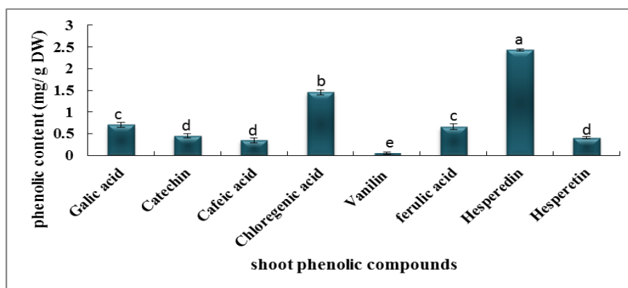
شکل ۶- انواع ترکیبات فنلی و فلاونوئیدی شناسایی شده شاخساره گیاه گیشدر ( Periploca aphylla ). داده‌ها میانگین سه تکرار ± SE است. براساس آزمون دانکن حروف متفاوت، نشان‌دهنده اختلاف معنی‌دار ( P \leq 0.05 ) هستند.
