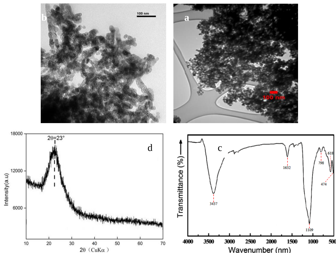
شکل ۱- (a) تصویر میکروسکوپ الکترونی روبشی (SEM)، (b) تصویر میکروسکوپ الکترونی عبوری (TEM)، (c) طیف‌سنجی تبدیل فوری مادون قرمز (FTIR)، (d) پراش اشعه ایکس (XRD) نانوذرات سیلیکون مورد استفاده در آزمایش
