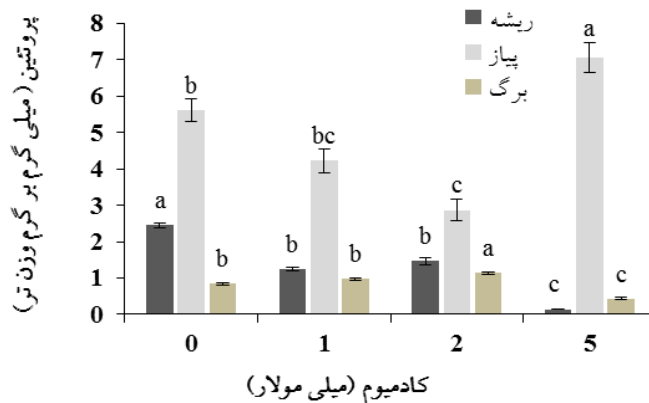
شکل ۵- مقدار پروتئین در گیاهچه‌های نرگس دو هفته پس از تیمار کادمیوم. اعداد میانگین ۴ تکرار \pm خطای استاندارد است. اختلافات معنی‌دار با اعداد متفاوت نشان داده شده است ( P < 0.05 ).
