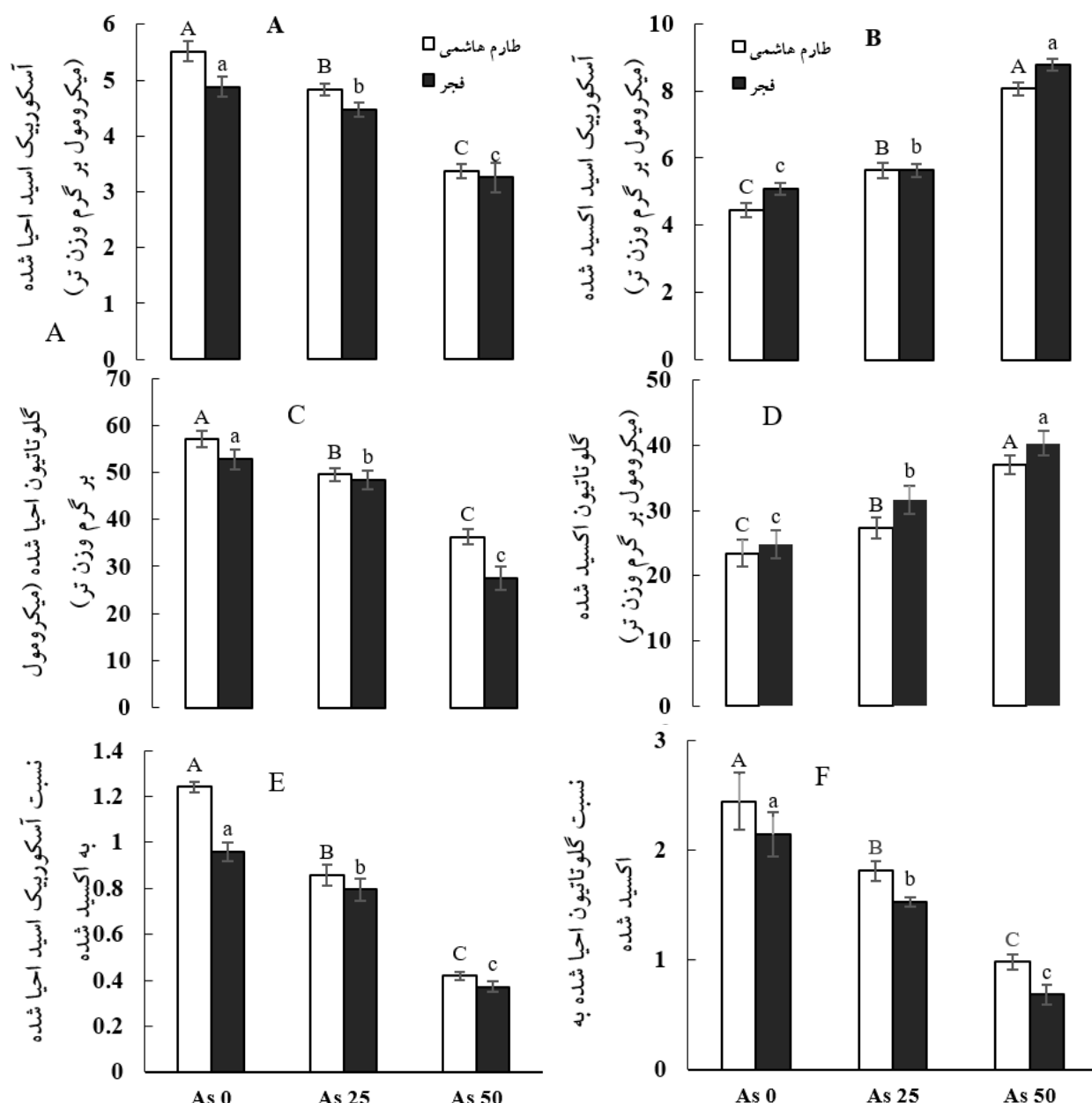
شکل ۳- تاثیر غلظت های مختلف آرسنیک (As، صفر، ۲۵ و ۵۰ میکرومولار) بر محتوای آسکوربیک اسید احیا شده (A)، آسکوربیک اسید اکسید شده (B)، گلو تاتیون احیا شده (C)، گلو تاتیون اکسید شده (D) و نسبت های آسکوربیک اسید احیا شده به اکسید شده (E) و گلو تاتیون احیا شده به اکسید شده (F) برگ دو رقم برنج طارم هاشمی و فجر. در هر رقم، میانگین های دارای حروف مشترک براساس آزمون LSD در سطح ۵ درصد تفاوت معنی داری با یکدیگر ندارند ( n = 4 \pm SD ).
