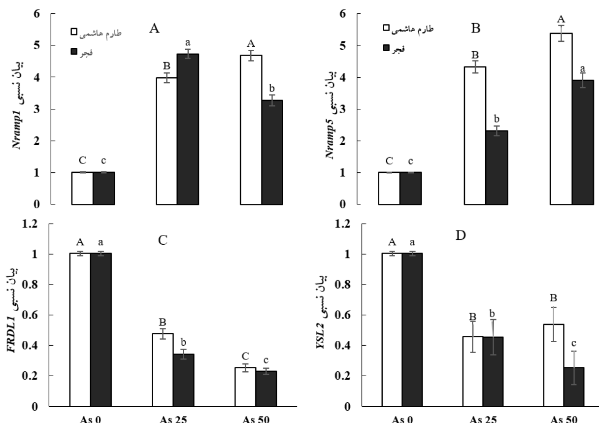
شکل ۵- تاثیر غلظت‌های مختلف آرسنیک (As، صفر، ۲۵ و ۵۰ میکرومولار) بر سطح بیان ژن‌های (A) Nrap1 ، (B) Nrap5 ، (C) FRDL1 و (D) YSL2 ریشه دو رقم برنج طارم هاشمی و فجر. در هر رقم، میانگین‌های دارای حروف مشترک براساس آزمون LSD در سطح ۵ درصد تفاوت معنی‌داری با یکدیگر ندارند ( n = 4 \pm SD ).
