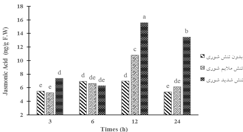
شکل ۳- محتوای هورمون جاسمونیک اسید در شرایط بدون تنش، تنش ملایم و تنش شدید (به ترتیب صفر، ۲۵۰ و ۶۰۰ میلی مولار کلرید سدیم) در زمان‌های ۳، ۶، ۱۲ و ۲۴ ساعت پس از اعمال تنش شوری. حروف مشابه نشان‌دهنده عدم وجود اختلاف معنی‌دار بین تیمارها براساس آزمون دانکن در سطح احتمال ۵ درصد است.
