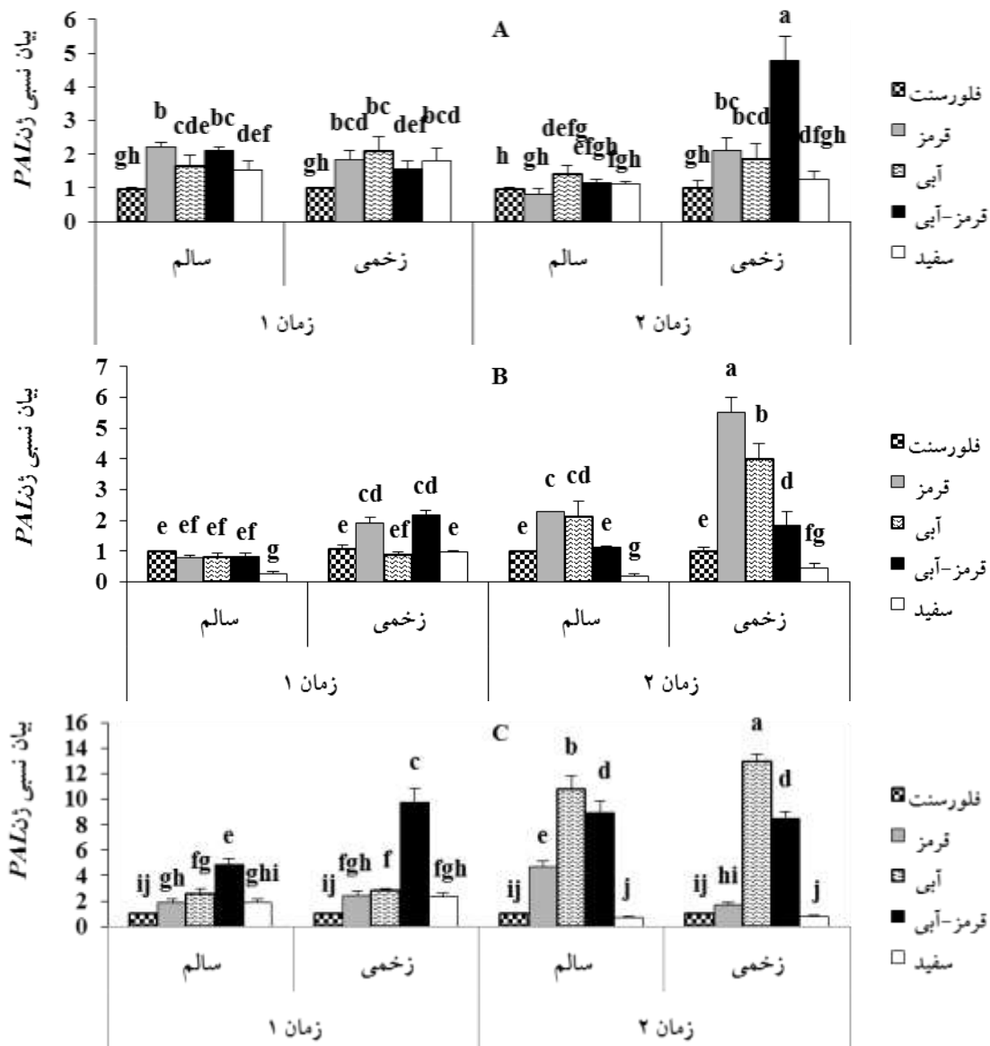
شکل ۶- تأثیر کیفیت نور، زخم و زمان نوردهی بر میزان بیان نسبی ژن PAL در برگ گیاه A. thaliana (A) ۲ ساعت، (B) ۲۴ ساعت و (C) ۱ هفته پس از ایجاد زخم. (حروف غیر یکسان بیانگر اختلاف معنی دار میانگین‌ها در سطح ۰/۰۵ آزمون LSD است).
