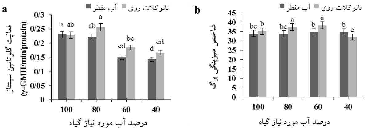
شکل ۲- اثرات متقابل تیمارهای آبیاری و محلول پاشی نانوکلات روی بر فعالیت گلوتامین سینتتاز (a) و شاخص سبزیگی برگ (b) سویا. میانگین‌های دارای حداقل یک حرف مشترک اختلاف معنی‌داری در سطح احتمال ۵ درصد با آزمون دانکن ندارند. میله‌های عمودی نشان‌دهنده انحراف معیار است.
