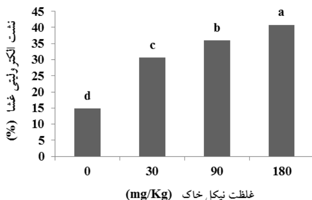
شکل ۳- مقایسه میانگین نشست الکترونی غشا در سطوح مختلف تیمار نیکل گیاهچه‌های فسکیوی بلند. حروف متفاوت بیانگر اختلاف معنی‌دار در سطح ۰/۰۵ است.
