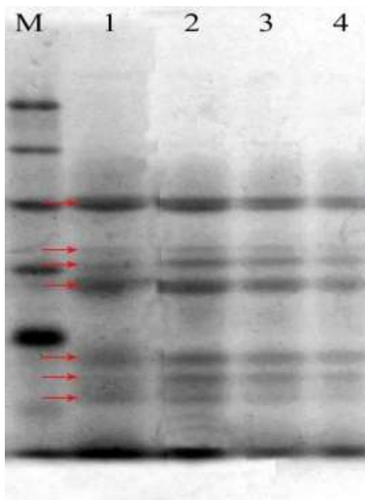
شکل ۸- مقایسه نیمرخ الکتروفورزی پروتئین‌های بذر در گروه شاهد و تحت تیمار غلظت‌های مختلف کادمیوم. M: مارکر پروتئینی، ۱، ۲، ۳ و ۴ به ترتیب باندهای پروتئینی بذرهای گروه شاهد، تحت تیمار ۷۵، ۱۵۰، ۲۲۵ میلی‌گرم بر لیتر کادمیوم. پیکان‌ها اختلاف در باندهای پروتئینی بین تیمارهای مختلف را نشان می‌دهند.
