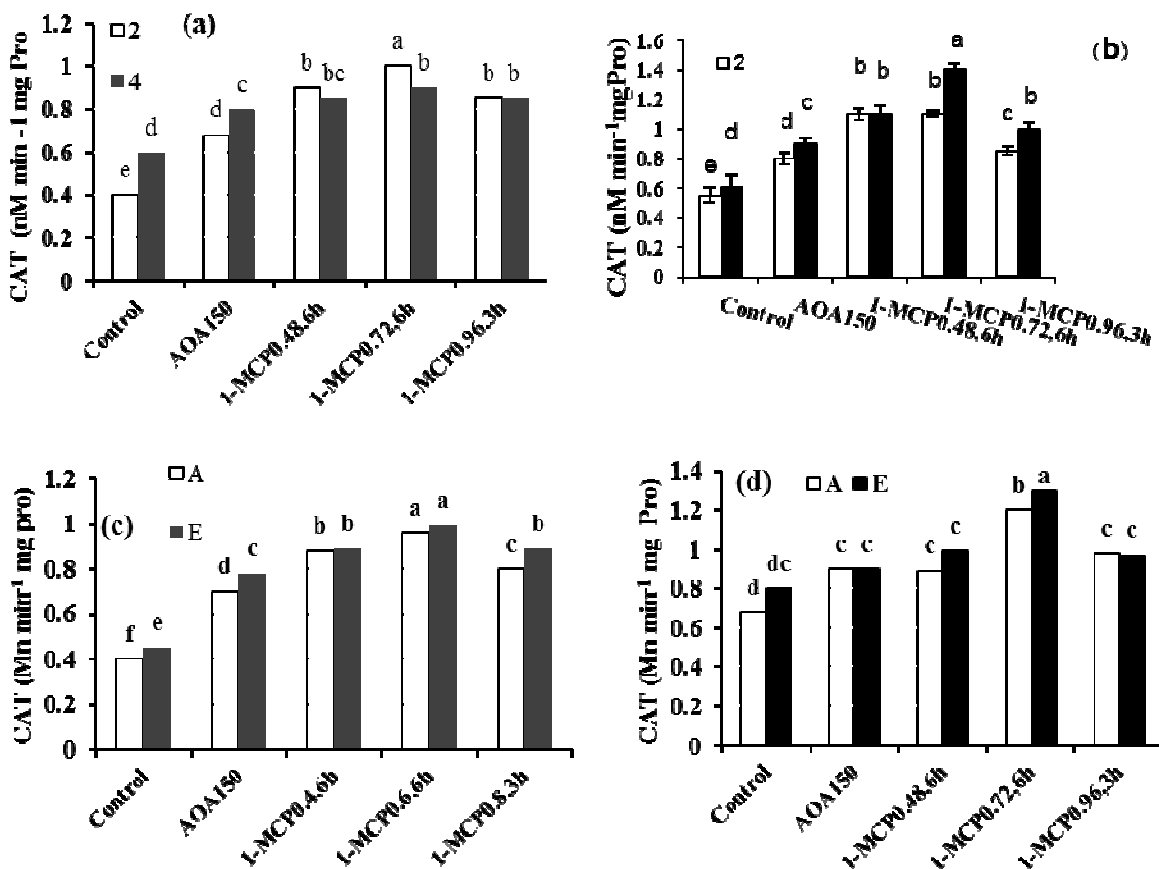
شکل ۵- تاثیر تیمارهای شیمیایی و دمای ۲ (□) و ۴ (■) درجه سانتی‌گراد بر فعالیت آنزیم کاتالاز (CAT) در روز اول (a) و سوم (b) تاثیر تیمارهای شیمیایی و رقم (■ Erueka و □ Aragon) بر فعالیت آنزیم کاتالاز در روز اول (c) و سوم (d) بعد از اتمام دوره انبارداری خشک. حروف مشترک بیانگر عدم اختلاف معنی‌دار بر اساس آزمون LSD می‌باشد.
