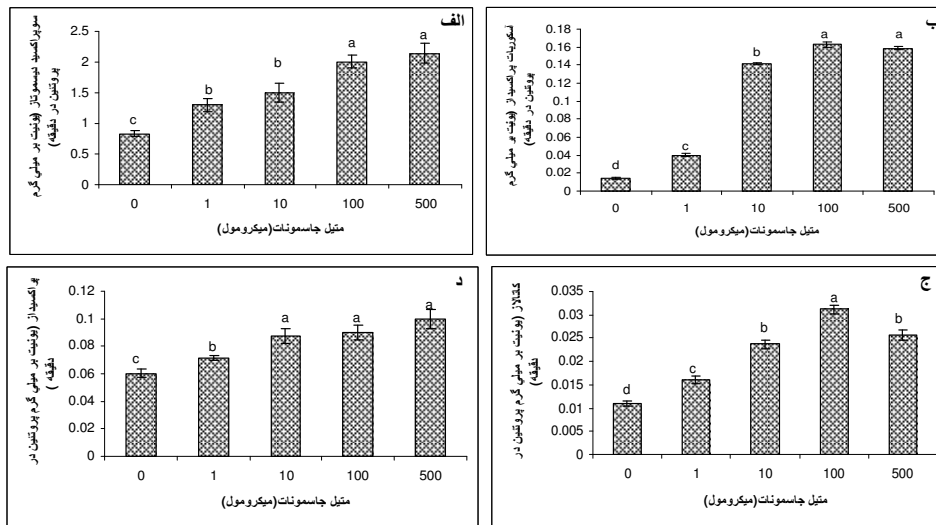
نمودار ۳- اثر میتیل جاسمونات بر فعالیت آنزیم‌های سوپر اکسید دیسموتاز (الف)، آسکوربات پراکسیداز (ب) کاتالاز (ج)، و پراکسیداز (د) در گیاه سویا در مرحله رویشی (مقادیر میانگین ۳ تکرار می باشد و حروف یکسان بیانگر عدم اختلاف معنی دار با استفاده از آزمون دانکن می باشد).
