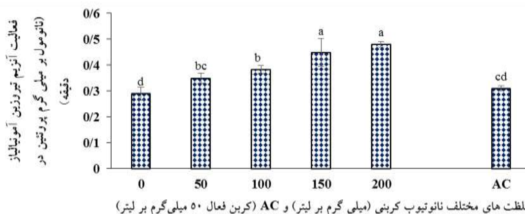
شکل ۱۳- تأثیر غلظت های مختلف نانولوله کربنی و کربن فعال بر فعالیت آنزیم تیروزین آمونیاپاز گیاه ریحان. مقادیر، میانگین سه تکرار \pm SE است و حروف غیر مشابه ستون ها معنی دار بودن میانگین داده ها براساس آزمون دانکن ( P < 0.05 ) را نشان می دهد.
