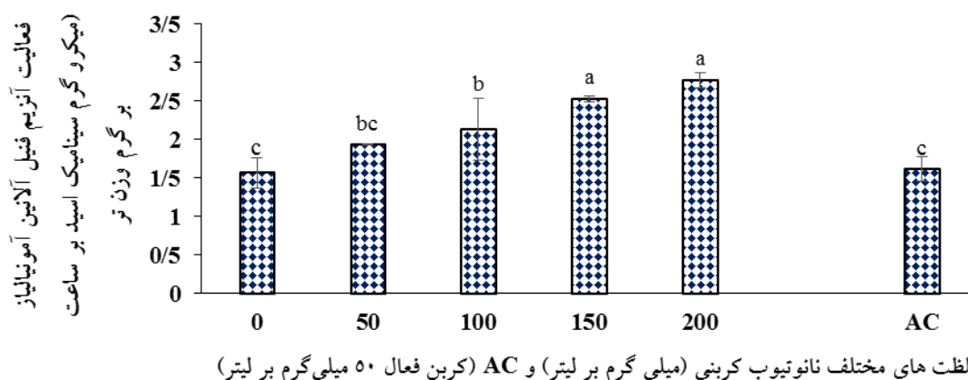
شکل ۱۲- تأثیر غلظت های مختلف نانولوله کربنی و کربن فعال بر فعالیت آنزیم فنیل آلانین آمونیاپاز گیاه ریحان. مقادیر، میانگین سه تکرار \pm SE است و حروف غیرمشابه ستون ها معنی دار بودن میانگین داده ها براساس آزمون دانکن ( P < 0.05 ) را نشان می دهد.
