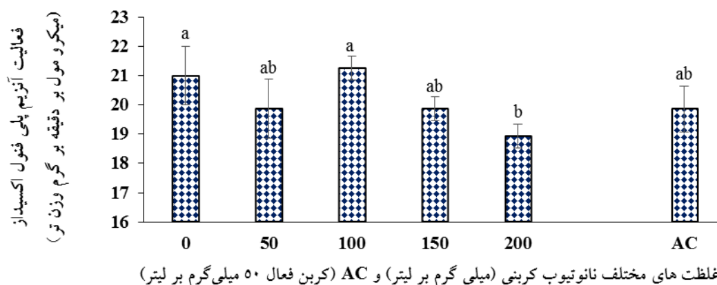
شکل ۱۱- تأثیر غلظت های مختلف نانولوله کربنی و کربن فعال بر فعالیت آنزیم پلی فنول اکسیداز گیاه ریحان. مقادیر، میانگین سه تکرار \pm SE است و حروف غیرمشابه ستون ها معنی دار بودن میانگین داده ها براساس آزمون دانکن ( P < 0.05 ) را نشان می دهد.
