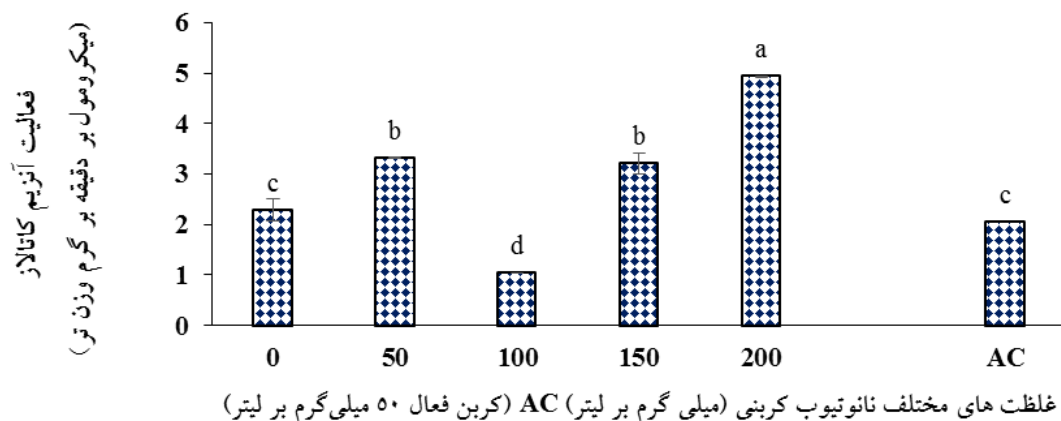
شکل ۹- تأثیر غلظت‌های مختلف نانولوله کربنی و کربن فعال بر فعالیت آنزیم کاتالاز گیاه ریحان. مقادیر، میانگین سه تکرار \pm SE است و حروف غیرمشابه ستون‌ها، معنی‌دار بودن میانگین داده‌ها براساس آزمون دانکن ( P < 0.05 ) را نشان می‌دهد.
